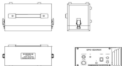
エポサーチ発信器(旧型)
